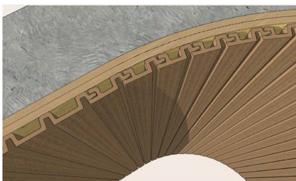
Vertikale Installation auf gewölbter, konkaver Wand mit Mini-Radius von 1 m
